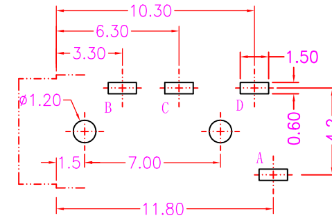
印制板开孔示意图
